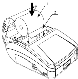
Рисунок 2. Заправка бумаги
