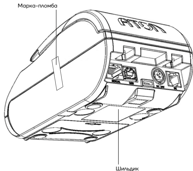
Рисунок 1. Расположение маркировки на корпусе ККТ
