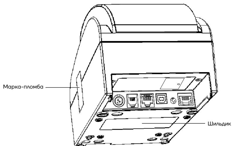
Рисунок 1. Расположение маркировки на корпусе ККТ
